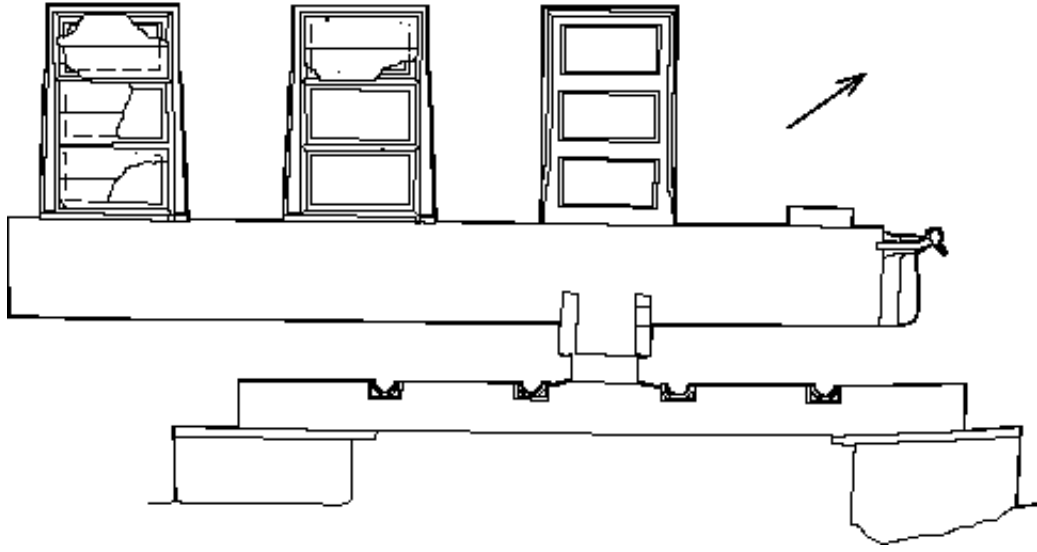
Resim 13: İran'dan I. Dareios'un mezar odasının planı (SCHMIDT 1970).
